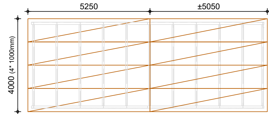
LEGPLAN VLOERPLATEN 8 stuks Vloerplaat 5.250x1.000x38 mm
